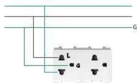
Sockets
